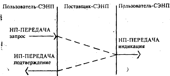
Рисунок 4 — Примитивы услуги НП-ПЕРЕДАЧА
