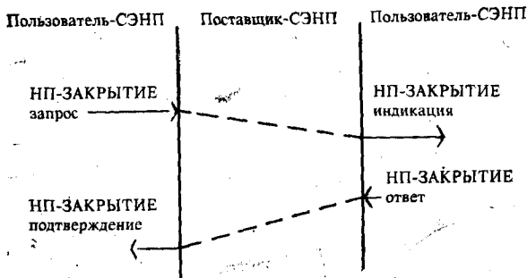
Рисунок 3 — Примитивы услуги НП-ЗАКРЫТИЕ
