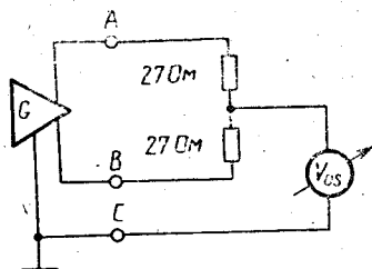
Рисунок 8 Измерение смещения напряжения
