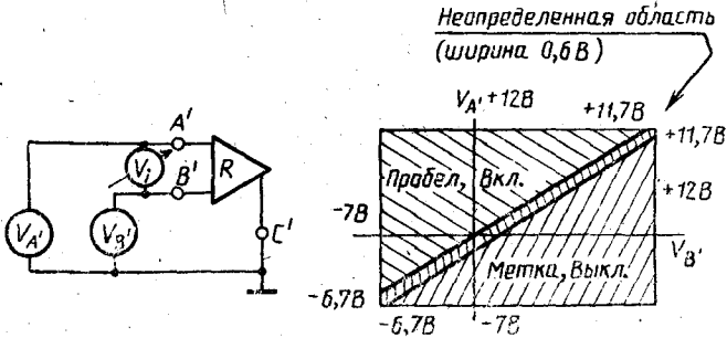
Рисунок 11 Диапазон входных напряжений
