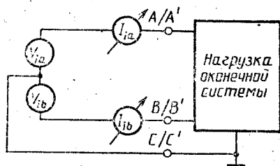
Рисунок 5 Измерение входного тока/напряжения
