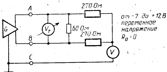
Рисунок 9 Измерение напряжения нагруженного выхода
