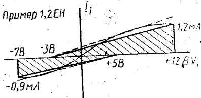
Рисунок 6 Определение значения ЕН
