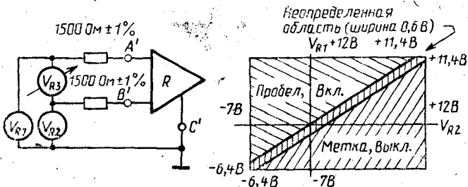
Рисунок 12 Измерение рассогласования на входе
