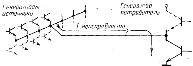
Рисунок 17 Соперничество генераторов с несколькими генераторами-источниками
