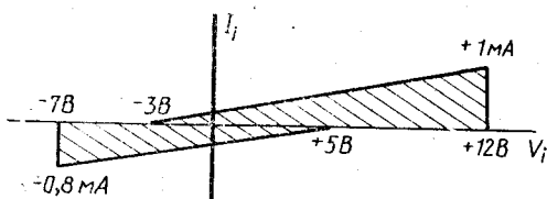
Рисунок 4 Ограничения тока 1,0 ЕН
