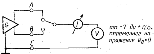
Рисунок 14 Проверка соперничества генераторов
