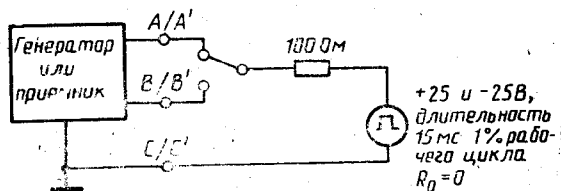
Рис. 15 Проверка переходного напряжения
