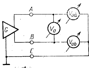
Рисунок 7 Измерение напряжения разомкнутой цепи
